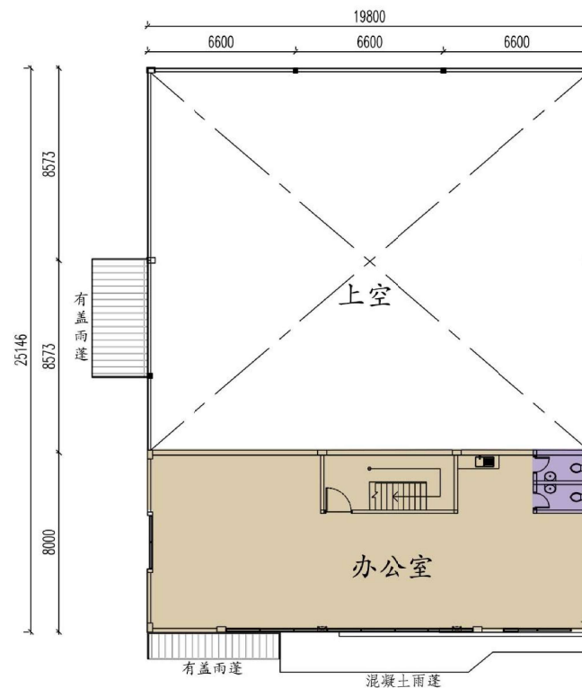
一楼平面图
